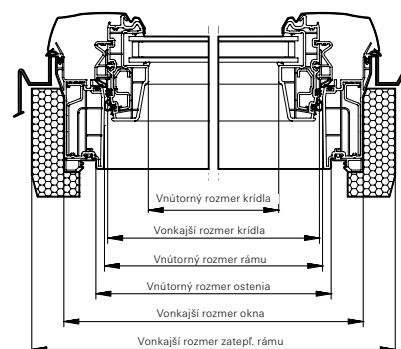
rez B-B
